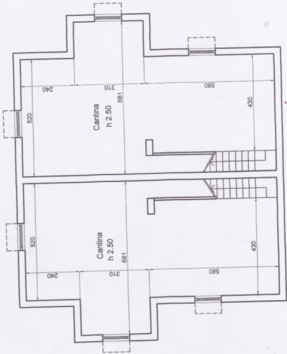
PIANTA PIANO Interrato 1:100
