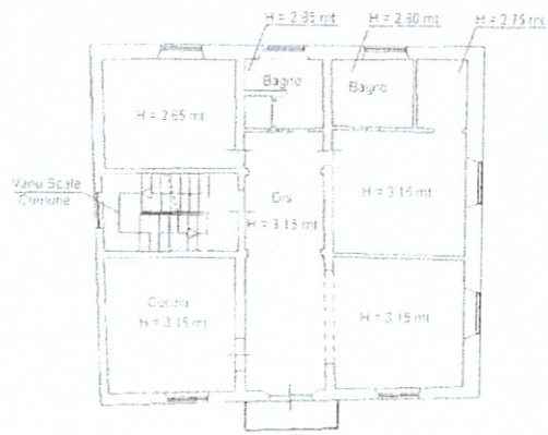
Piano Primo
