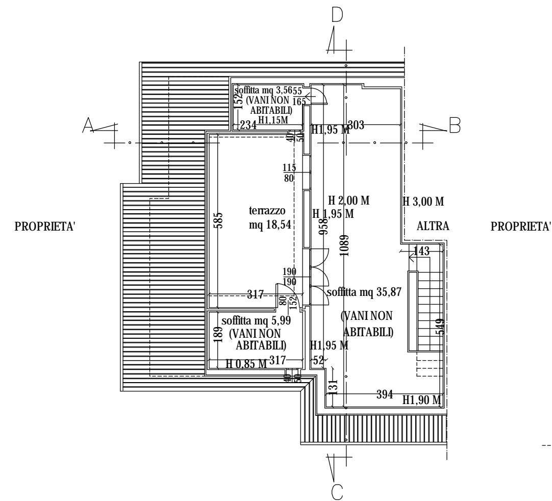
PIANTA PIANO SOTTOTETTO
