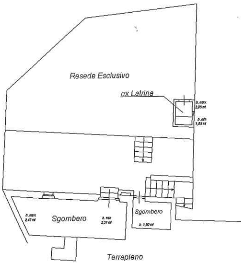
PIANO SOTTOSTRADA
