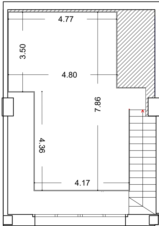
piano primo
