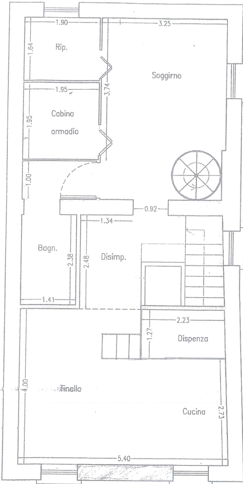
Pianta stato di progetto scala 1:50
