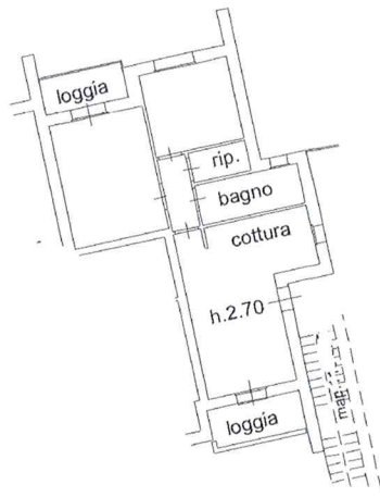
PIANO PRIMO
