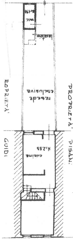
PIANO TERZO
