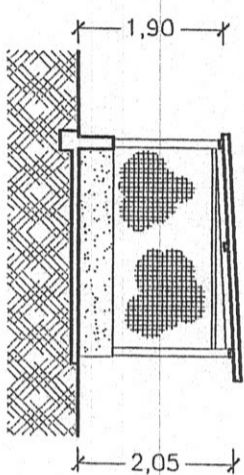
Sezione B-B'
