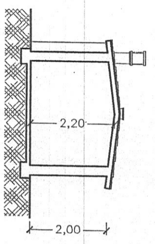
Sezione A-A'
