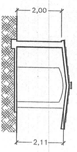
Sezione B-B'
