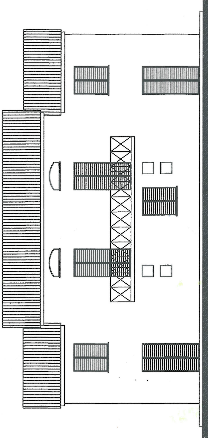
Prospetto Sud
