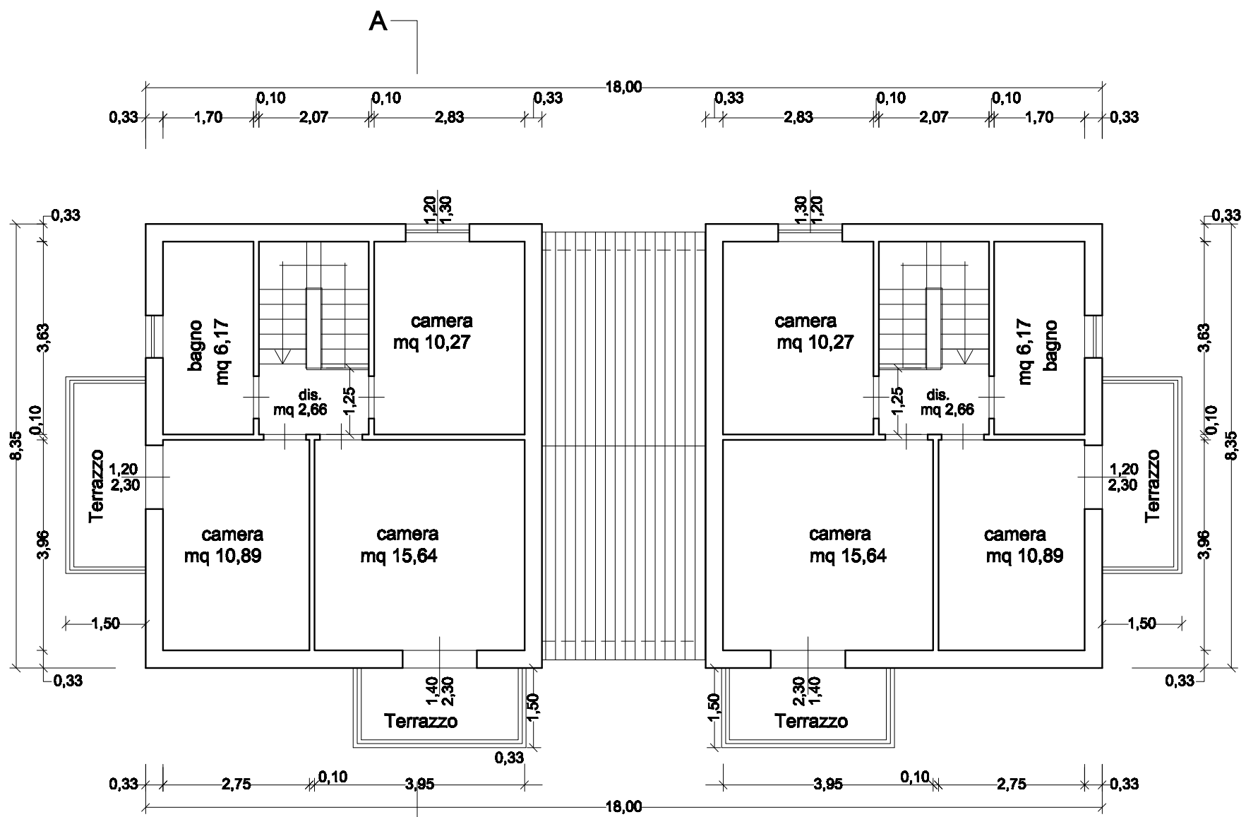
PIANO PRIMO
