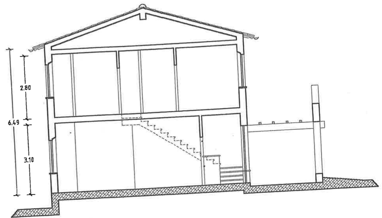
sezione
