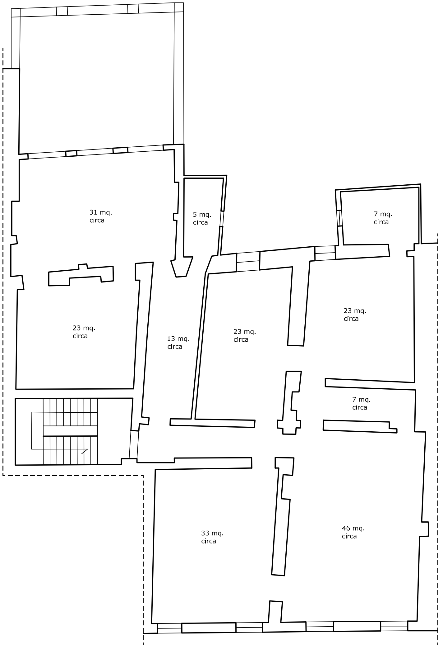
Stato attuale - scala 1:100
