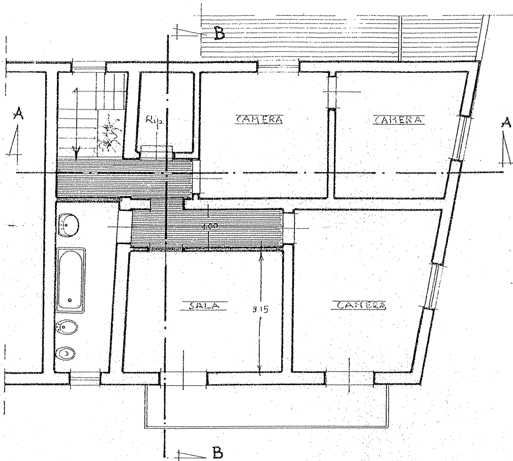
PIANTA 1° PIANO
