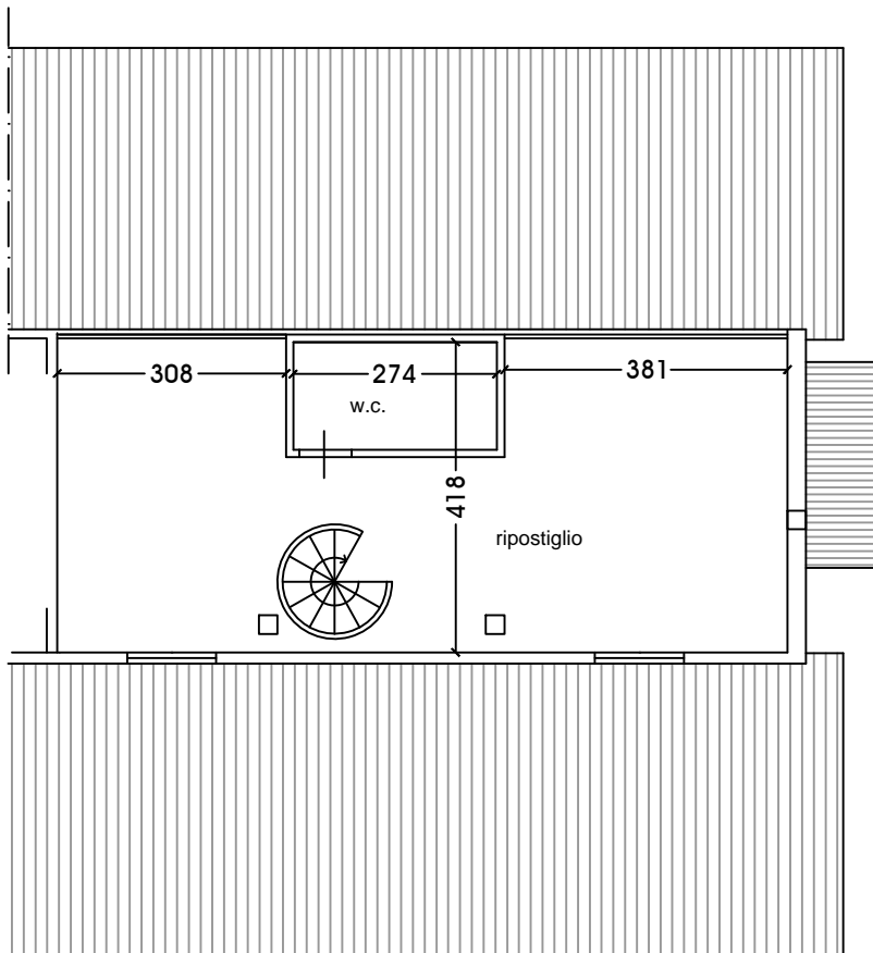
PIANTA SOTTOTETTO
