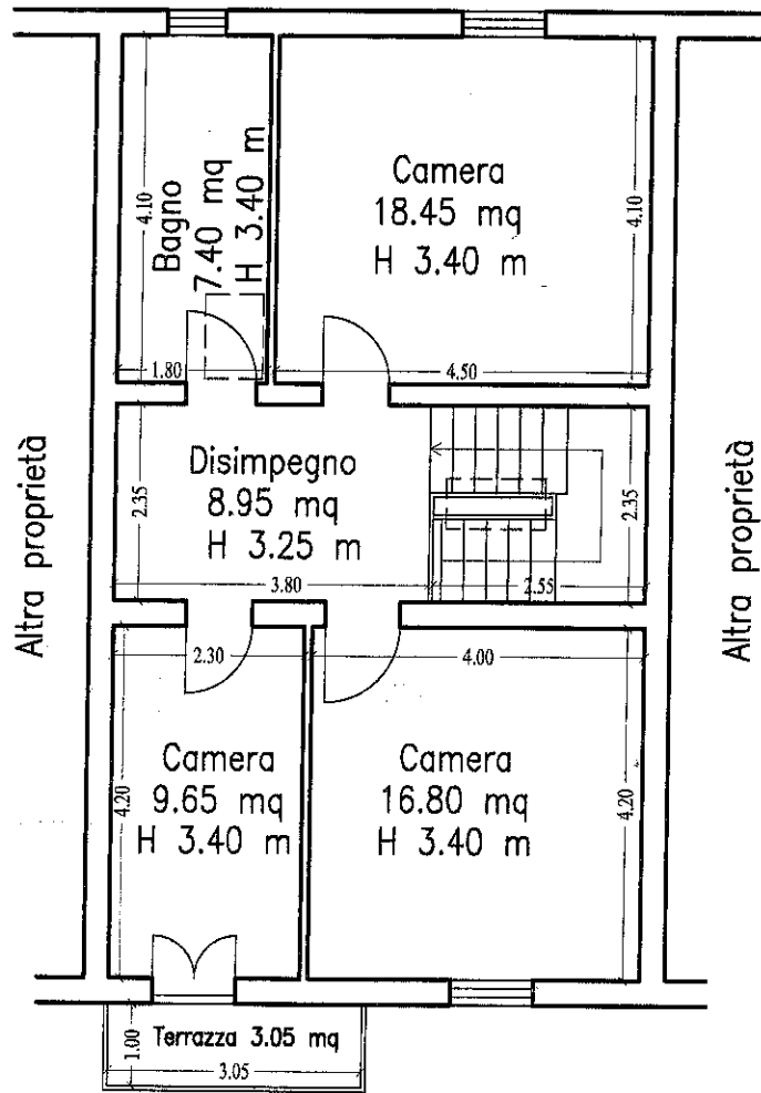
PIANO PRIMO
