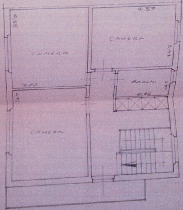
PIANTA PIANO PRIMO - 1/100
