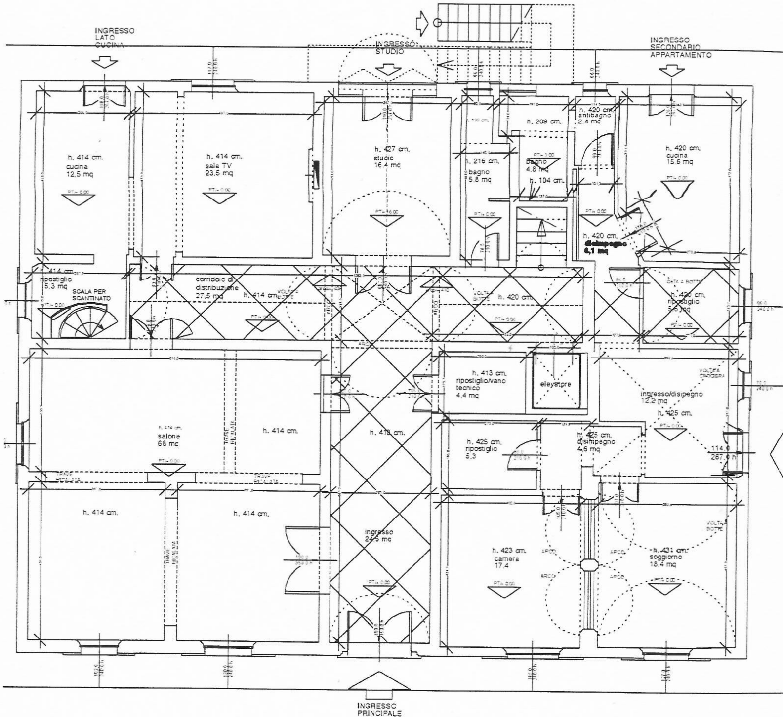
PIANTA PIANO TERRA STATO DI FATTO
